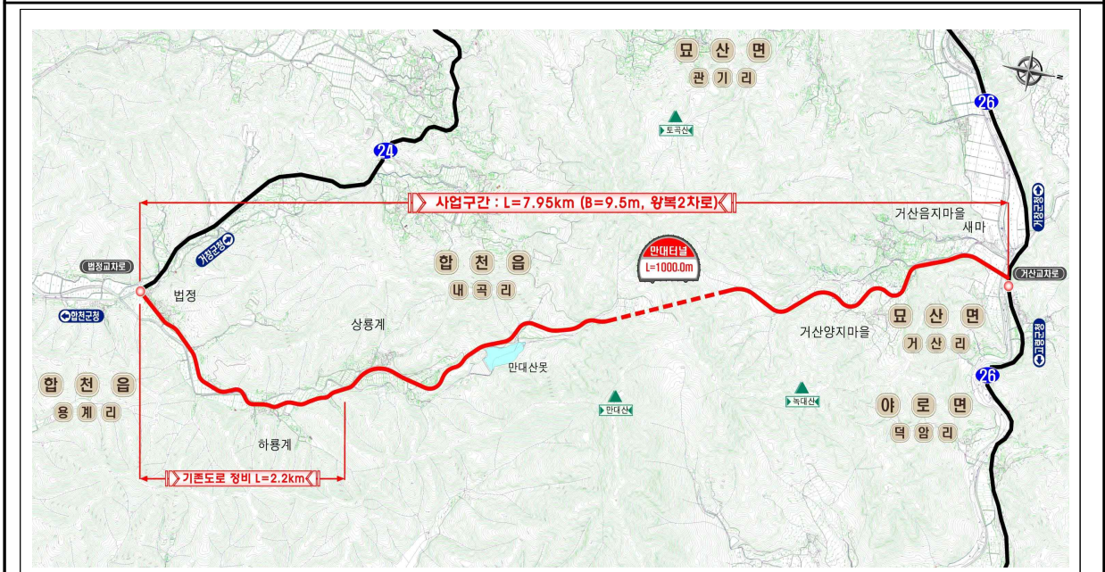
< 계획평면도 >
